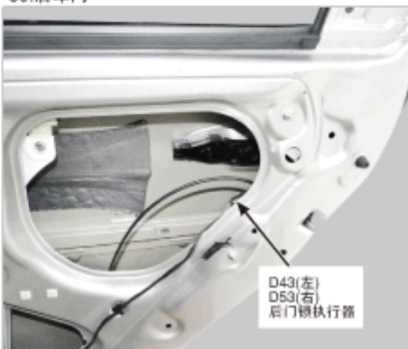
86.后车门
