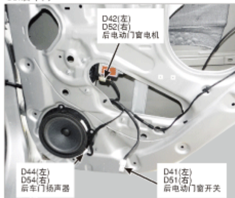
85.后车门
