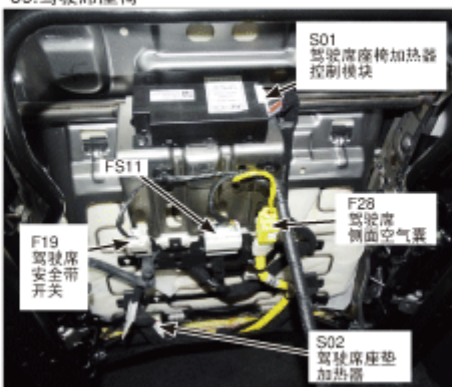
89.驾驶席座椅
