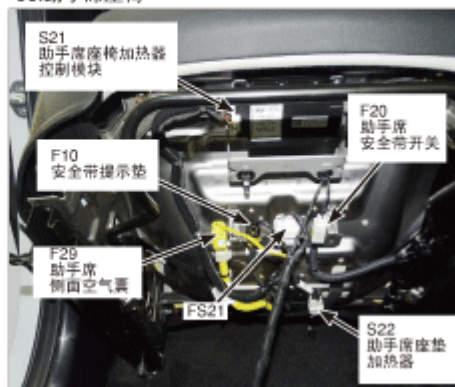
90.助手席座椅
